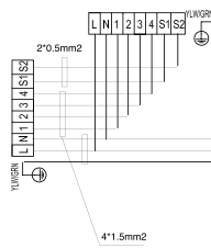
Модель LAC-24
