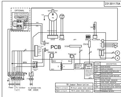
Схема для внутренних блоков (Модель LAC-24TC)
